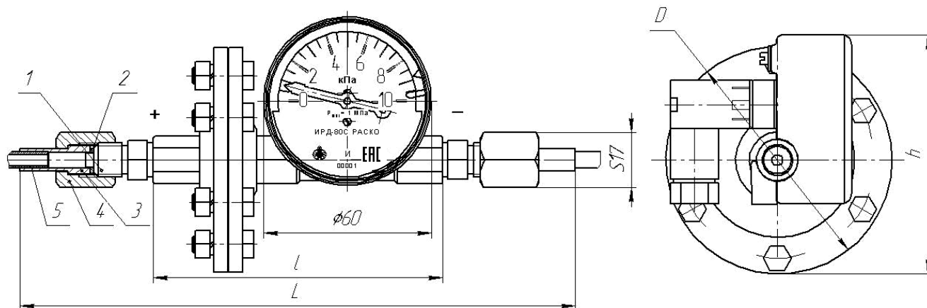
Рисунок Б.1 – Габаритные и присоединительные размеры индикатора с штуцерно-нипельным соединением
