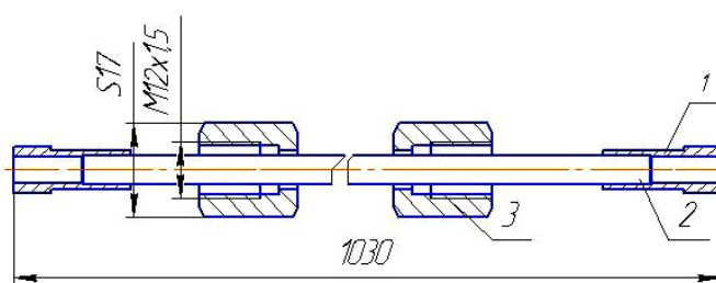
Рисунок Б.3 - Соединение с врезавшимся кольцом
