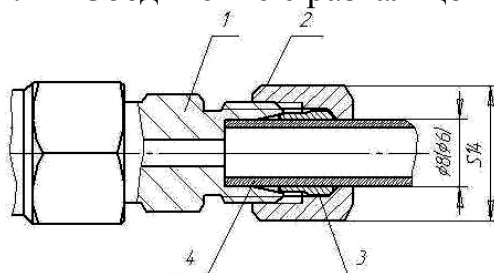
Рисунок Б.2 – Соединение с развальцовкой трубы
