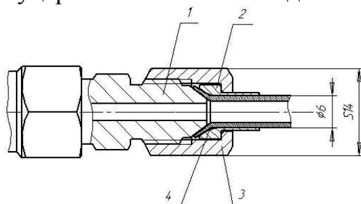
Рисунок Б.1 – Габаритные и присоединительные размеры индикатора с штуцерно-нипельным соединением
