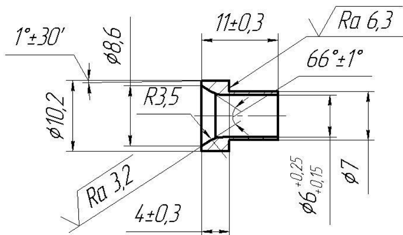
Рисунок Б.6 – Присоединительные размеры ниппеля
